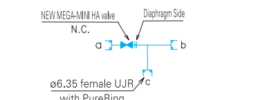
FPR-NSDTRO-721-6.35-2-316LP
