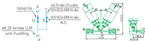
FBNSDV-721-6.35-2B3-316LP-BHJ
