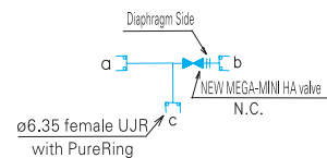
FPR-NSDTR-721-6.35-2-316LP
