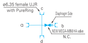
FPR-NSDXT-721-6.35-2-316LP
