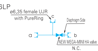
FPR-NSDTL-721-6.35-2-316LP
