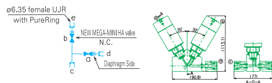
FBNSDV-721-6.35-2B3-316LP-BHI
