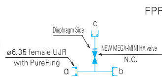
FPR-NSDTB-721-6.35-2-316LP
