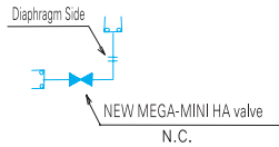
FPR-NSDCL-721-6.35-2-316LP
